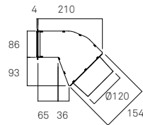
D1010 3 ВИХІДНИХ ОТВОРИ
