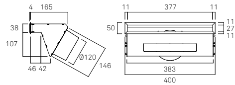
D1002 1 ВИХІДНИЙ ОТВІР (ВУЗЬКИЙ)
