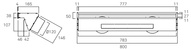
D1007 2 ВИХІДНИХ ОТВОРИ (ВУЗЬКИЙ)
