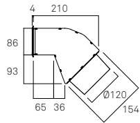
D1005 2 ВИХІДНИХ ОТВОРИ
